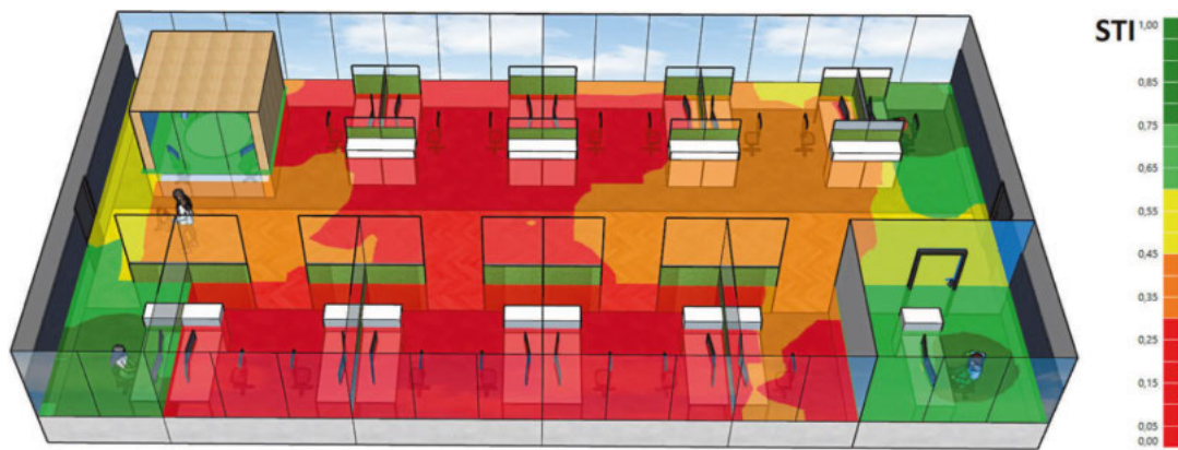
I Variante 3a: Sprachverständlichkeit; Hintergrundgeräusch = 45 dB(A) (z. B. Büro mit Besetzung und im typischen Betrieb); STI sinkt im Vergleich zu 35 dB(A) deutlich und reduziert dadurch u. U. das Ablenkungspotenzial über kurze und weitere Distanzen.
